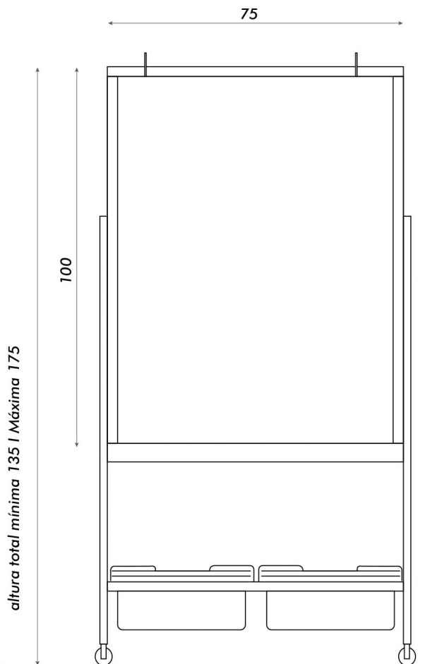
Dimensiones / Vista frontal
